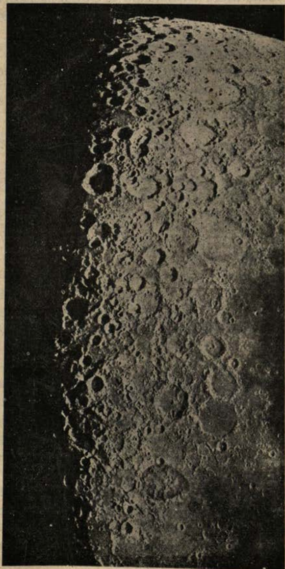
Какъ изглежда луната по краищата си. Чернитѣ петна сж трапчини, глѣбнатини, дупки, кратери, а бѣлитѣ точки и рѣбове сж върхове на планинитѣ.
