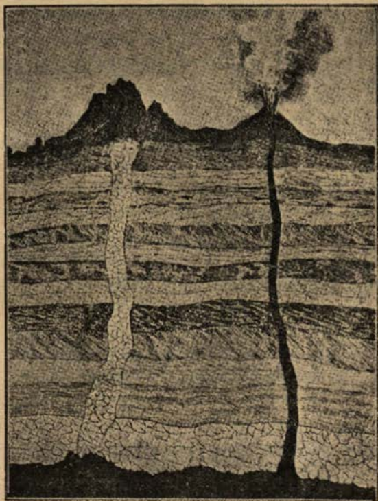
Разрѣзъ на земната кора. Отлѣво изгасналъ вулканъ; отдѣсно действащъ.
