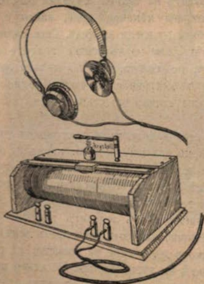
Малък радио-приемателъ.
