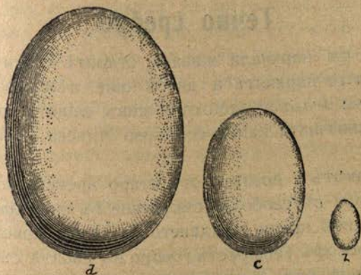
Обр. 3. А. Яйце отъ епиорнисъ, Б. отъ камилска птица, В. отъ кокошка
