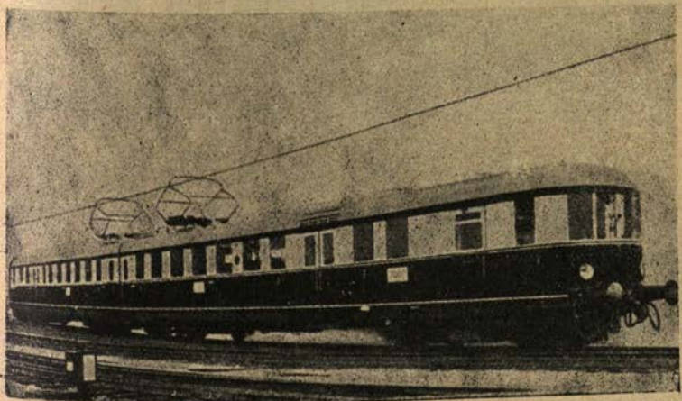
Електрически вагонъ отъ германскитѣ държавни желѣзници съ най-голѣма скоростъ 120 километра въ часъ
