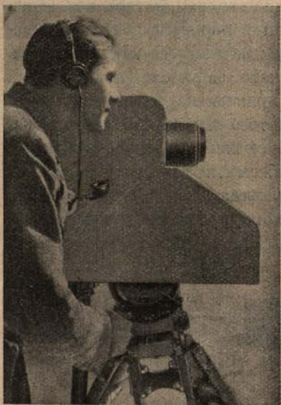
Телевизионна камера за снимане. (Телефункенъ)
