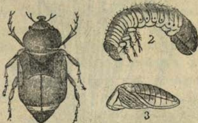
Житенъ бръмбаръ. — 2. Личинка 3. Какавида.
